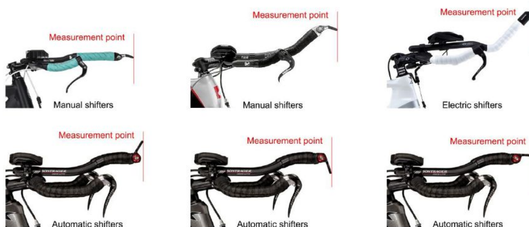
Figure 38 : Points de mesure de la distance horizontale depuis l'axe du boîtier de pédalier
