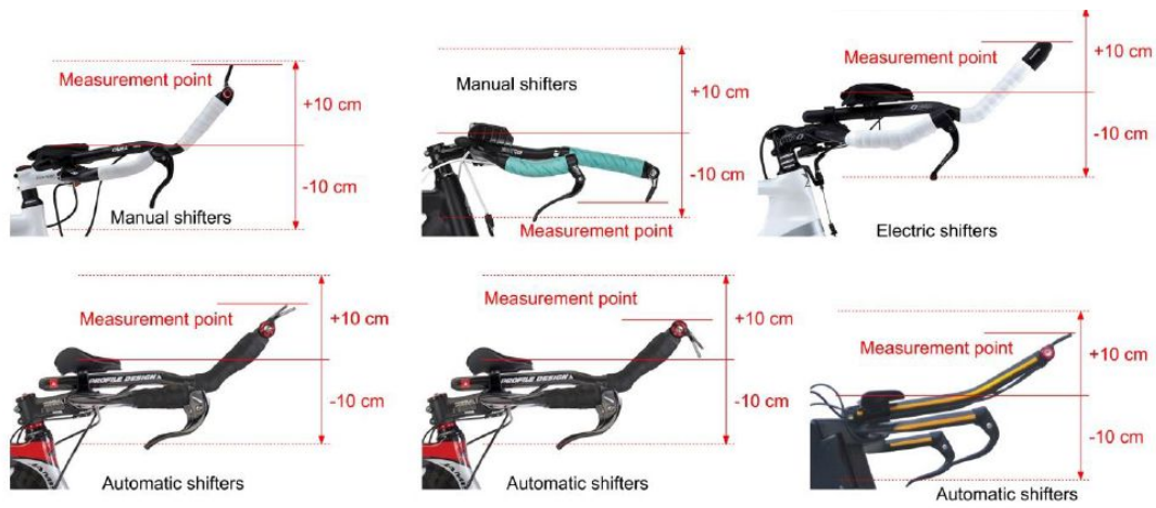
Figure 31 : Points de mesure des limites verticales des prolongateurs avec tous leurs accessoires
