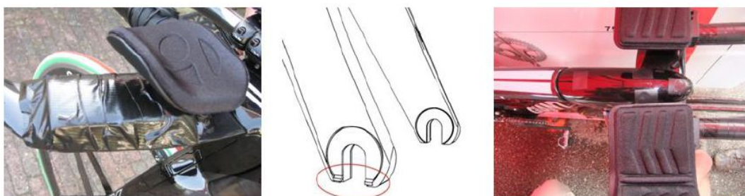
Figure 2 : Quelques exemples de modification du matériel interdit (ajout de tape, limage des ergots de fourche et recouvrement des vis du cadre et du guidon)
