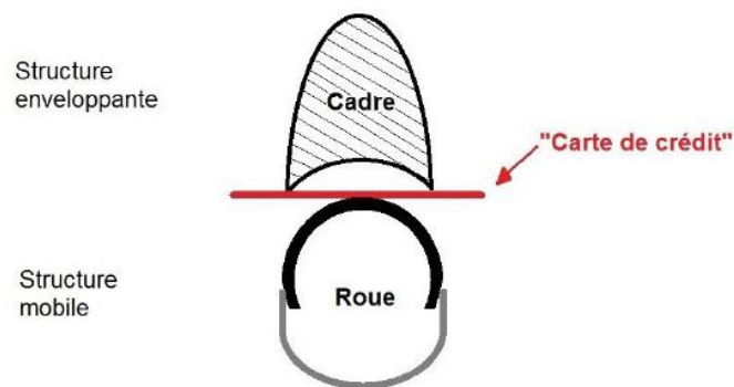
Figure 52 : Illustration du carénage des roues
