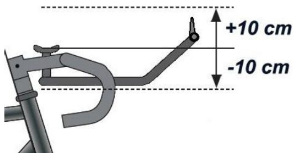
Figure 30 : Illustration des limites verticales des prolongateurs avec tous leurs accessoires
